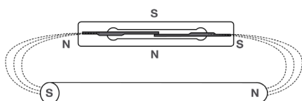
Flussverlauf Magnet-Reedkontakt
