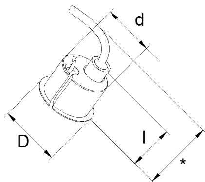
Magnetkontakt zum Einlassen *Mindesteinbautiefe
