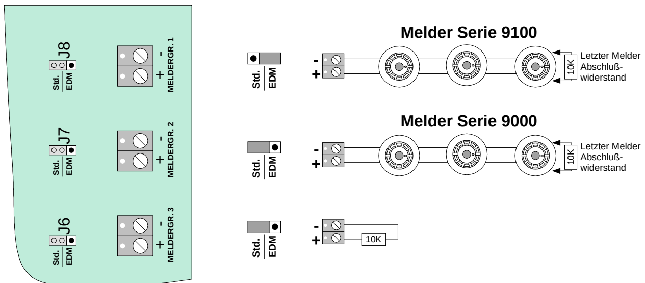
Abb. 25: Anschluss von Brandmeldern (Prinzipdarstellung)
