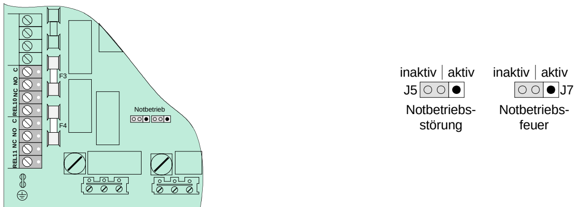
Abb. 33: Kodierbrücken zur Einstellung der Notbetriebsfunktion
