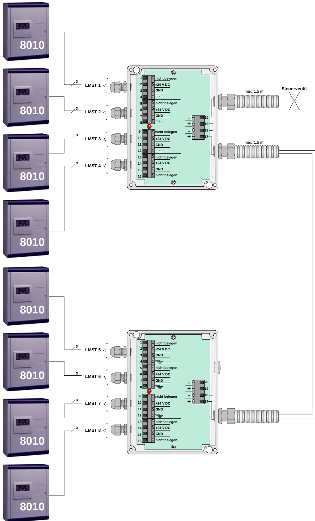
Abb. 40: Beispiel für die Anwendung der Mehrbereichssteuerung
