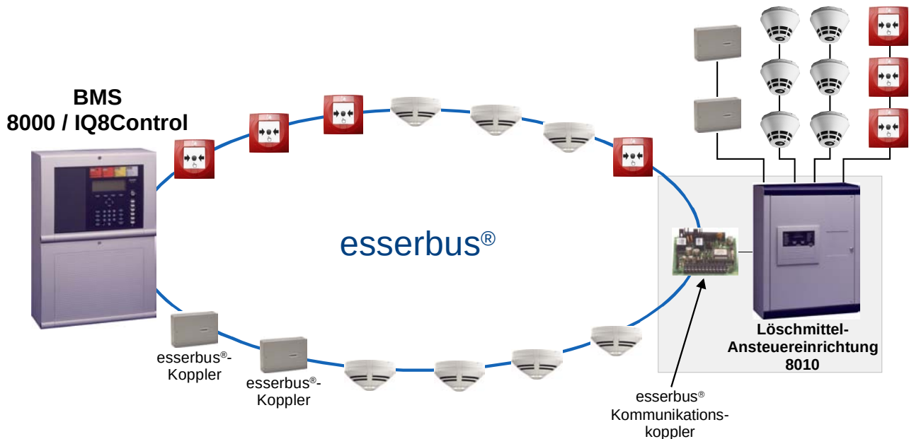
Abb. 39: Anschluss der Löschmittel-Ansteuereinrichtung 8010 an die Analog-Ringleitung
