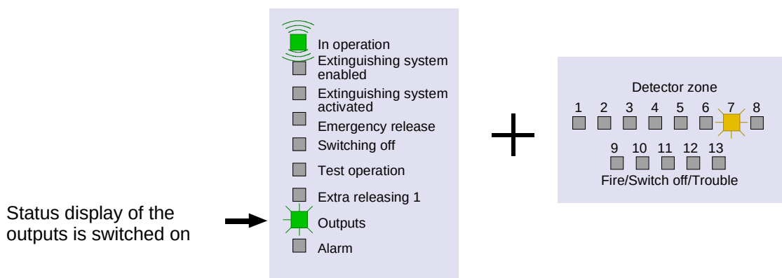
Fig. 3: Outputs displays
