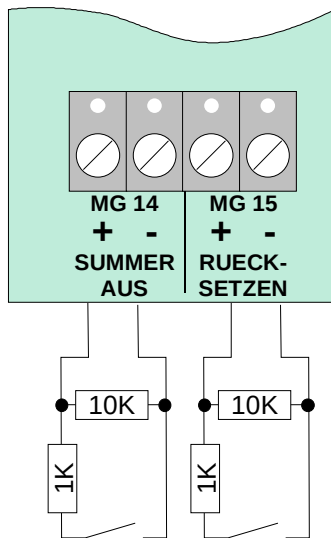
Abb. 27: Steuereingang MG14 und MG15
