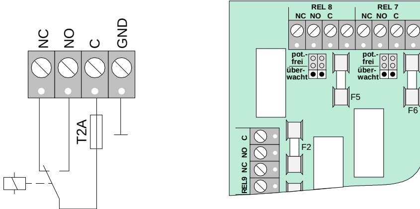
Abb. 31: Prinzipbeschaltung der Betriebsart "potentialfrei"
