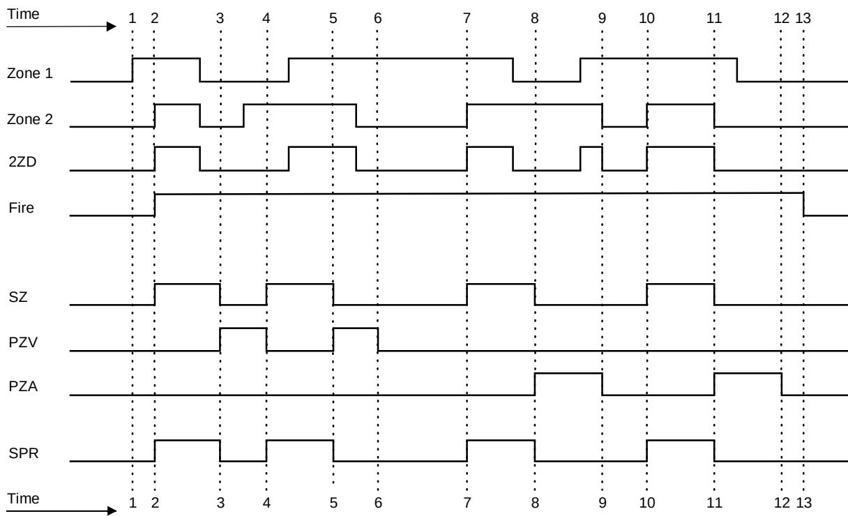
Fig. 37: Sequence diagram (AquaSafe)
