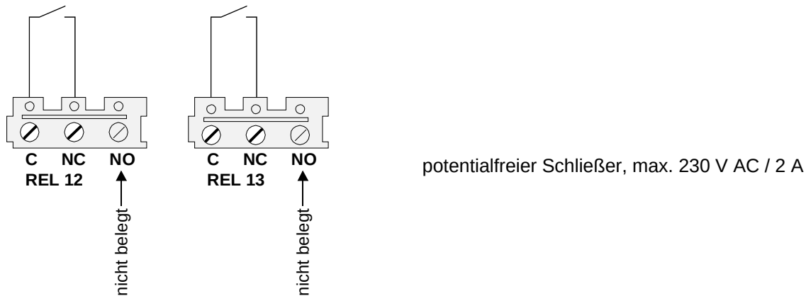
Abb. 29: Relais 12 und 13
