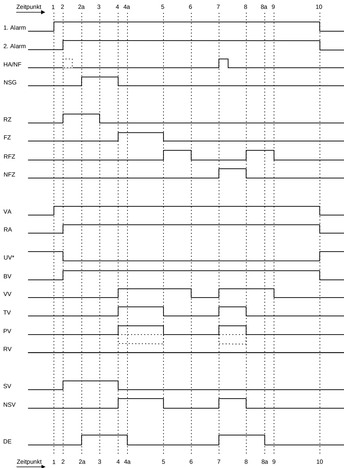
Abb. 36: Ablaufdiagramm (Löschmittelsteuerung)
