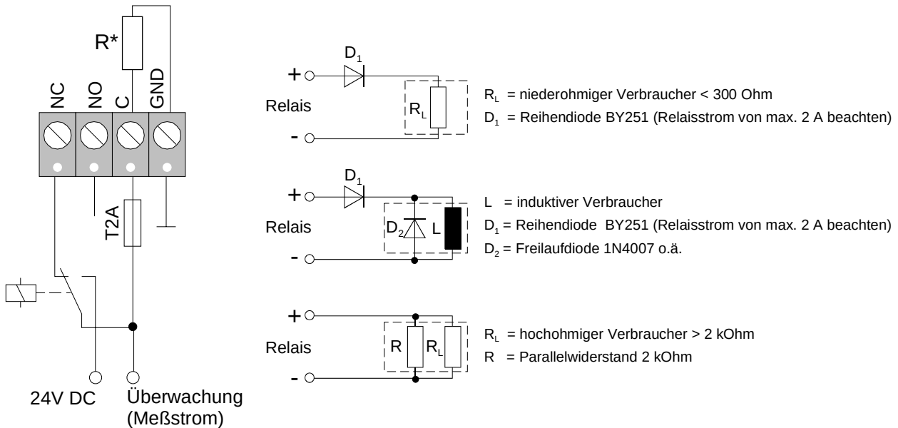
Abb. 32: Prinzipbeschaltung der Betriebsart plusschaltend / überwacht
