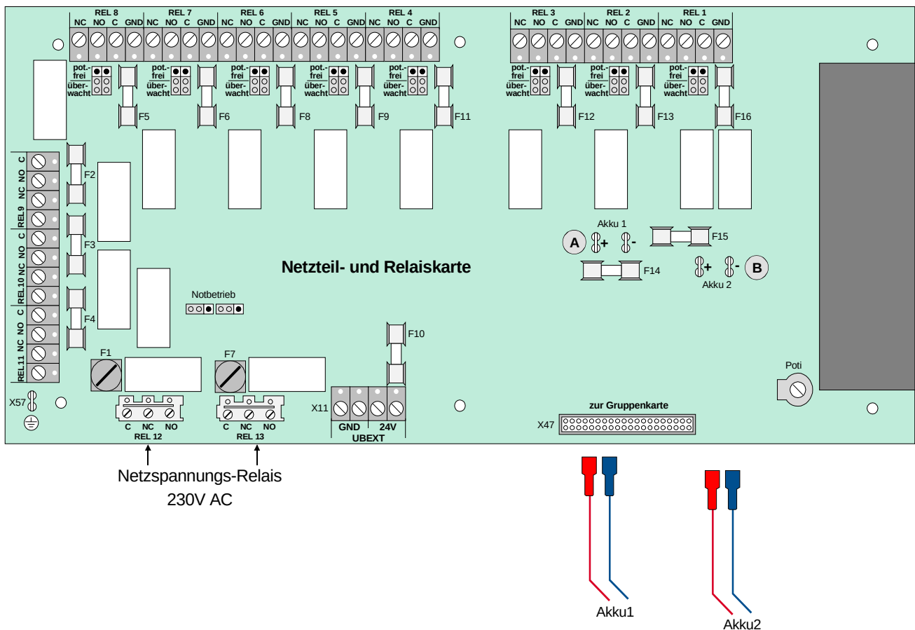
Abb. 28: Netzteil- und Relaiskarte / Lage der Baugruppen
