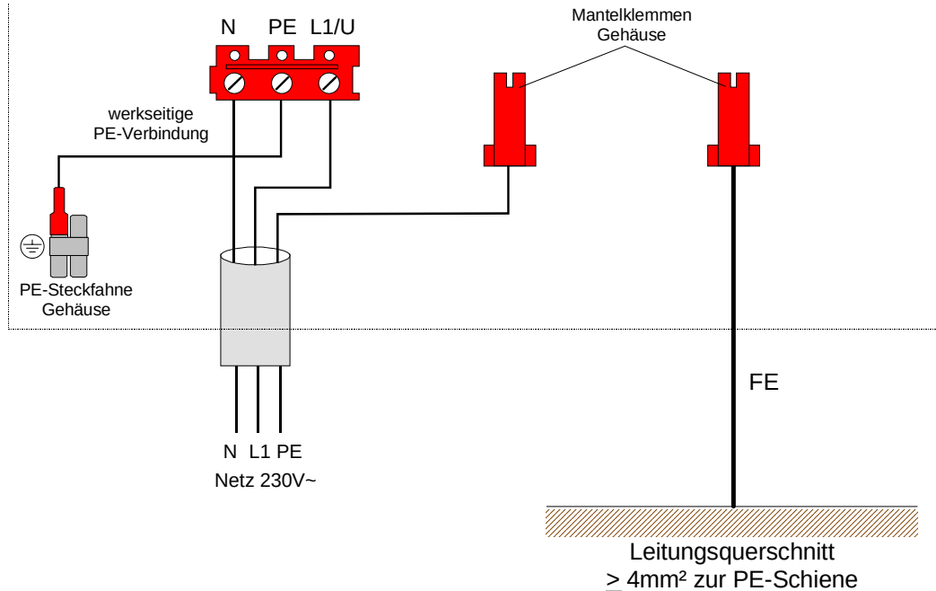
Abb. 21: Netzanschluss und Anschluss des Schutzleiters
