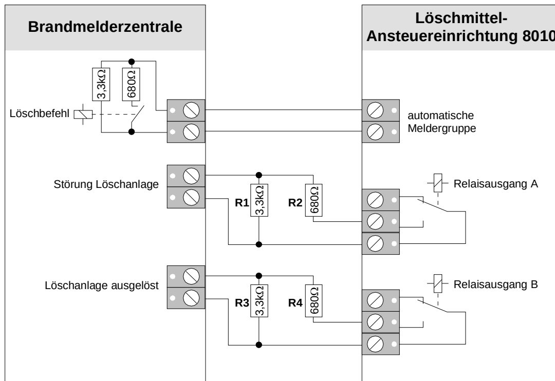
Abb. 34: Standardschnittstelle Löschen
