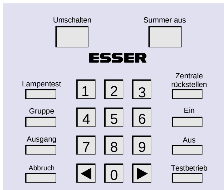
Abb. 6: Bedienfeldtastatur der Löschmittel-Ansteuereinrichtung 8010 - Serie 2
