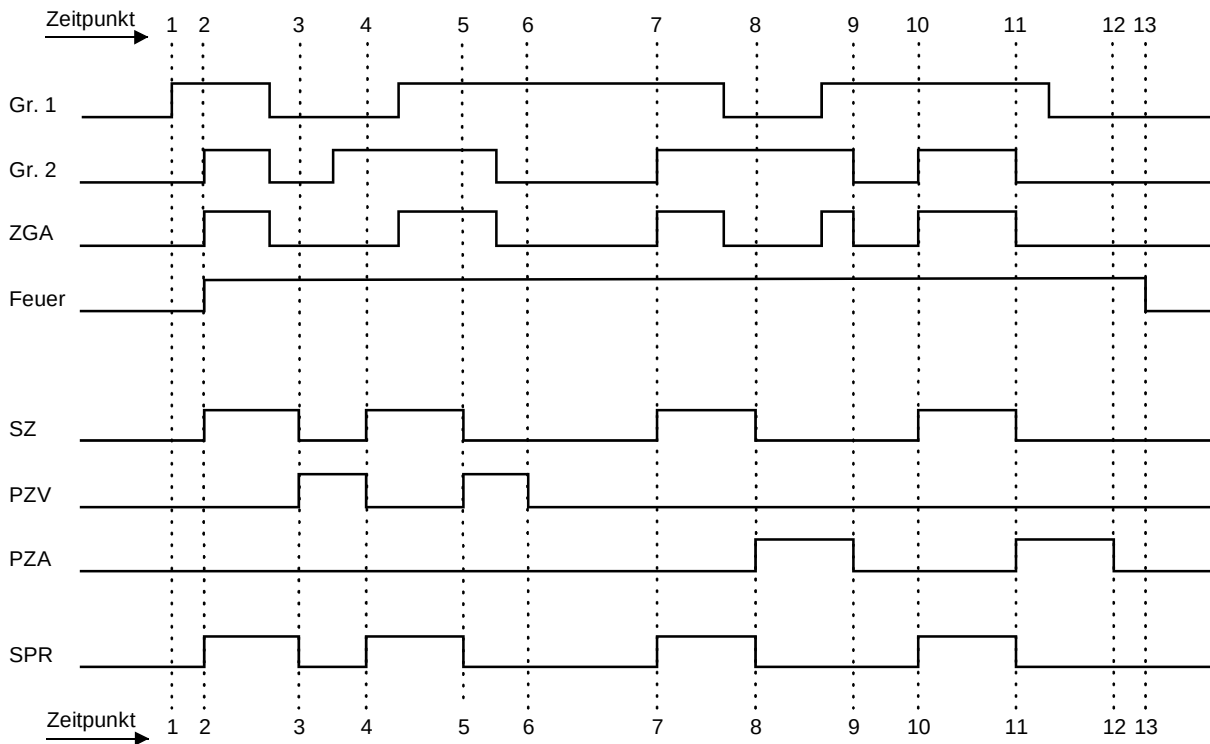
Abb. 37: Ablaufdiagramm (AquaSafe)
