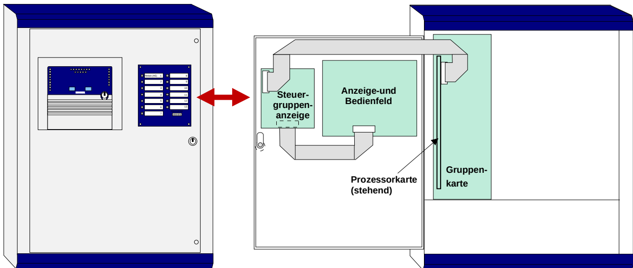
Abb. 35: Einbau der optionalen Anzeige für Steuergruppen
