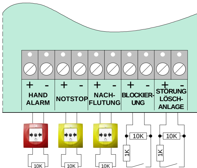
Abb. 26: Beschaltung der technischen Gruppen
