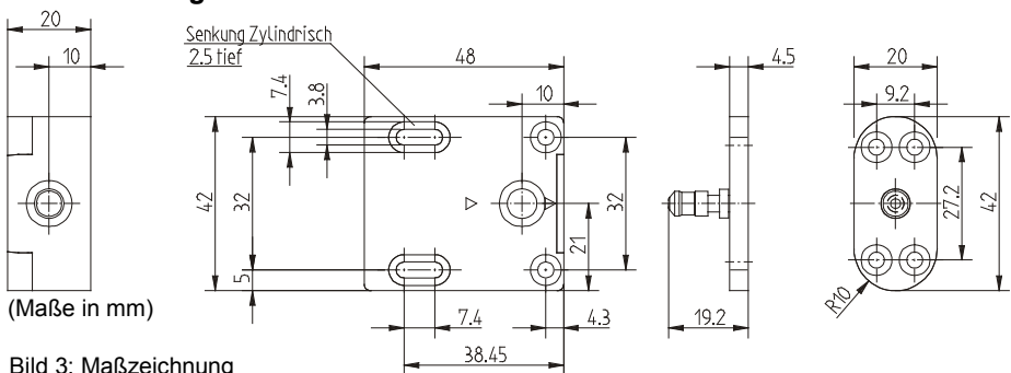
Bild 3: Maßzeichnung
