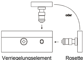
Bild 1: Verriegelungsprinzip
