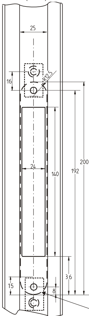
Türrahmen (Türöffner) Door Frame (strike)
