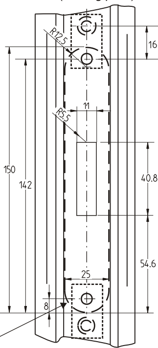
Türblatt (Schließblech) Door Leaf (Striking plate)
