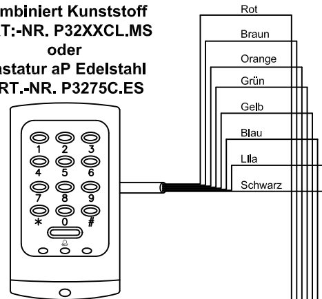
Tastatur / Leser aP kombiniert Kunststoff ART.-NR. P32XXCL.MS oder Tastatur aP Edelstahl ART.-NR. P3275C.ES
