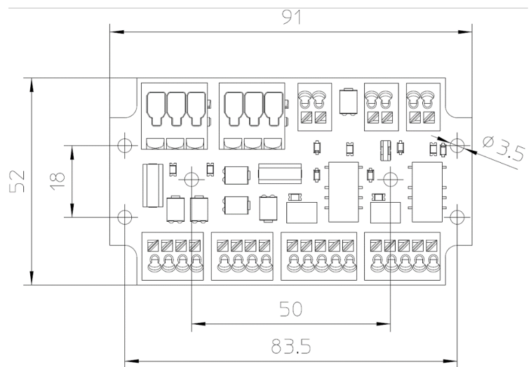
Abmessungen
