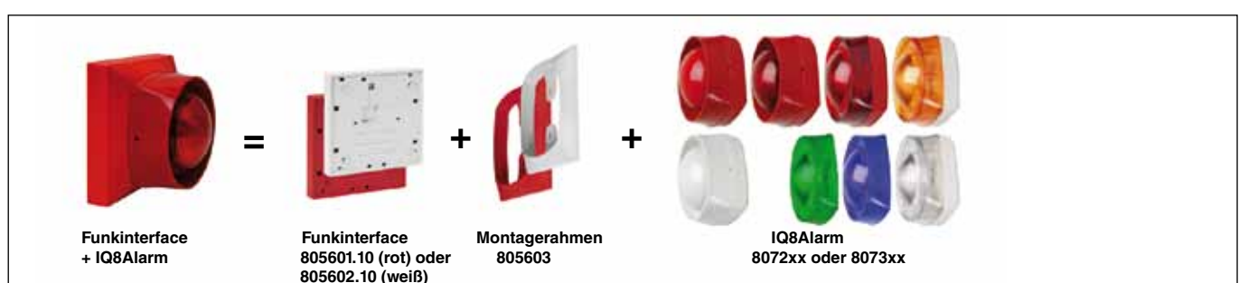
Aufbau Funkinterface mit IQ8Alarm
